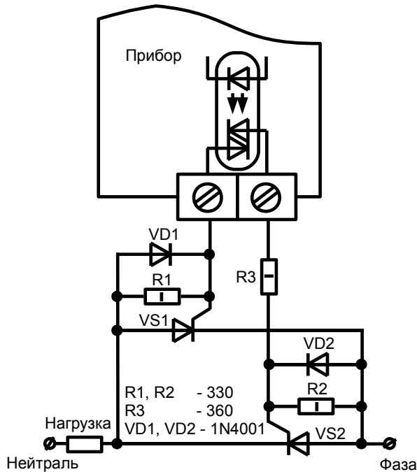
г) пример использования симисторной оптопары для управления силовыми тиристорами
